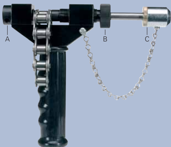
Bolzenlöser
